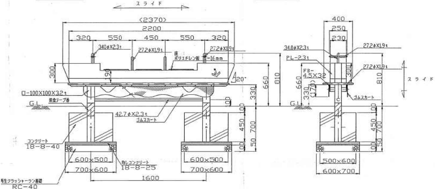
立面図
