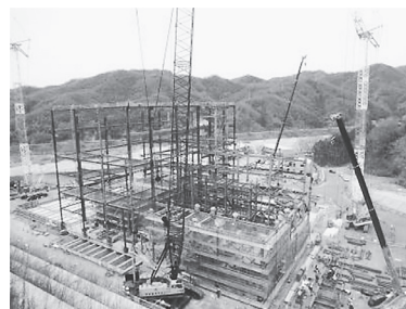
施設鉄筋建方工事（平成29年3月）
