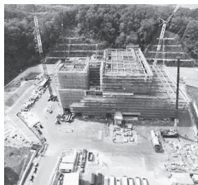
外壁建込工事(平成29年8月)
