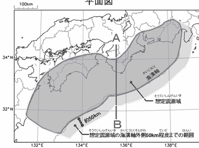
へいめんず 平面図
