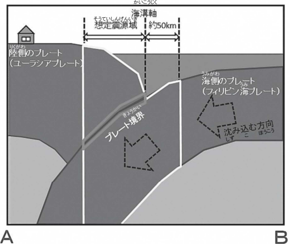
だんめんず 断面図
