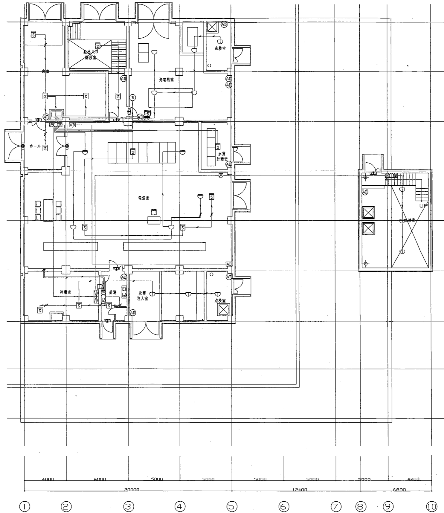
1階平面図
