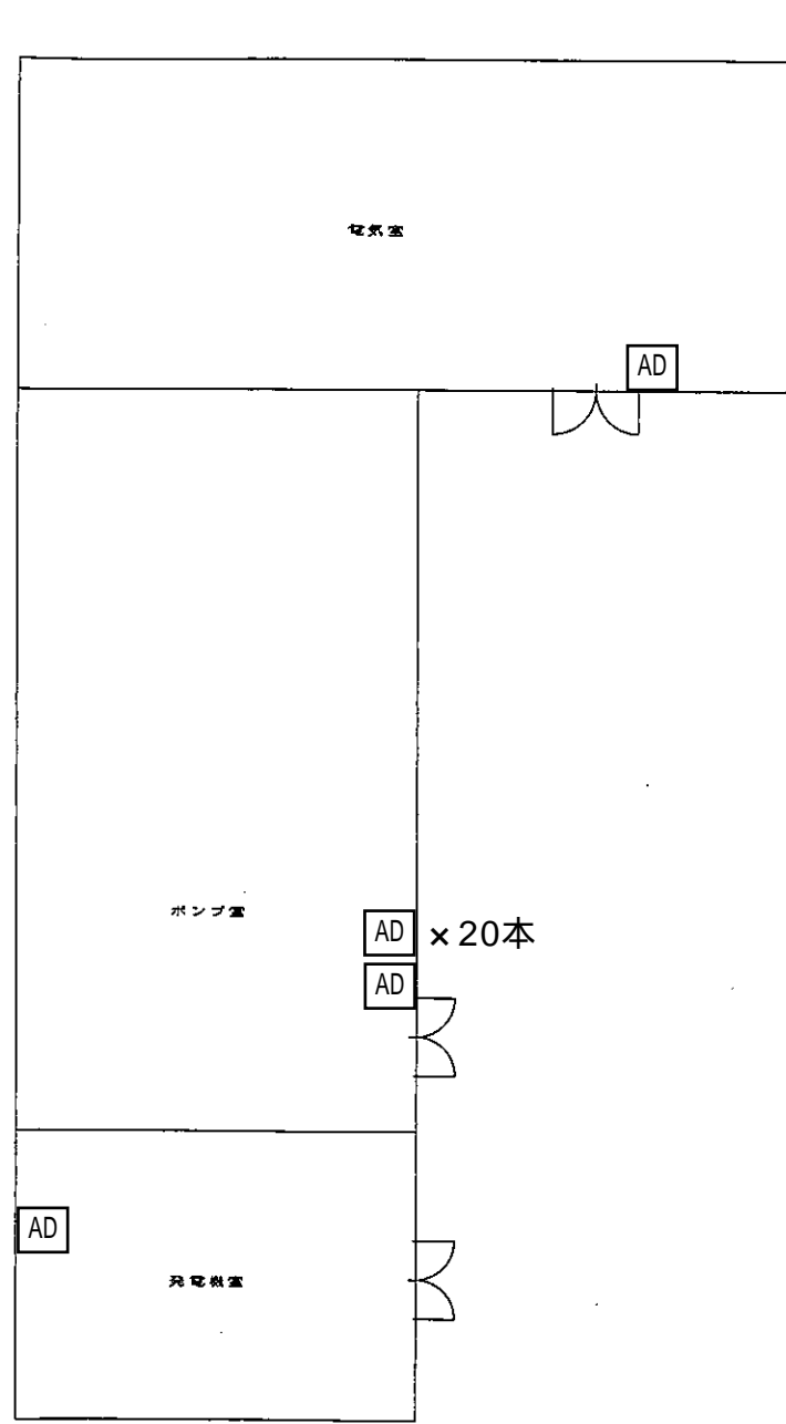
祝園受水場 電気室平面図 S=1/100
