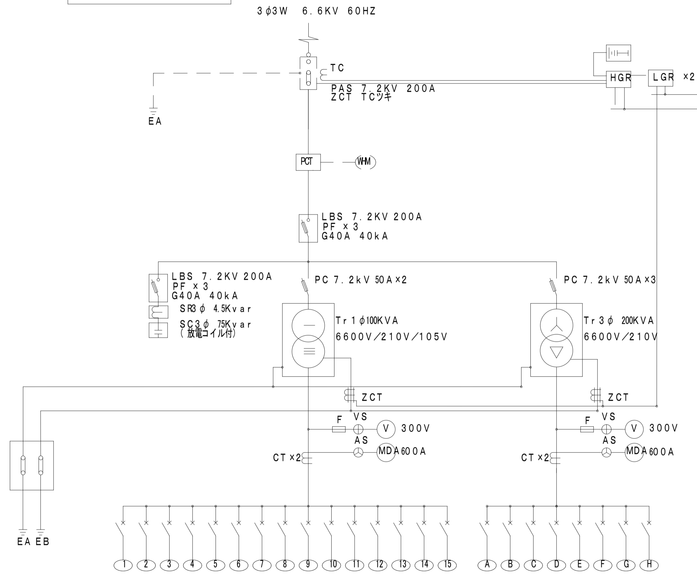
新設キュービクル参考姿図
