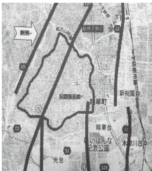
政府活用の活断層図
